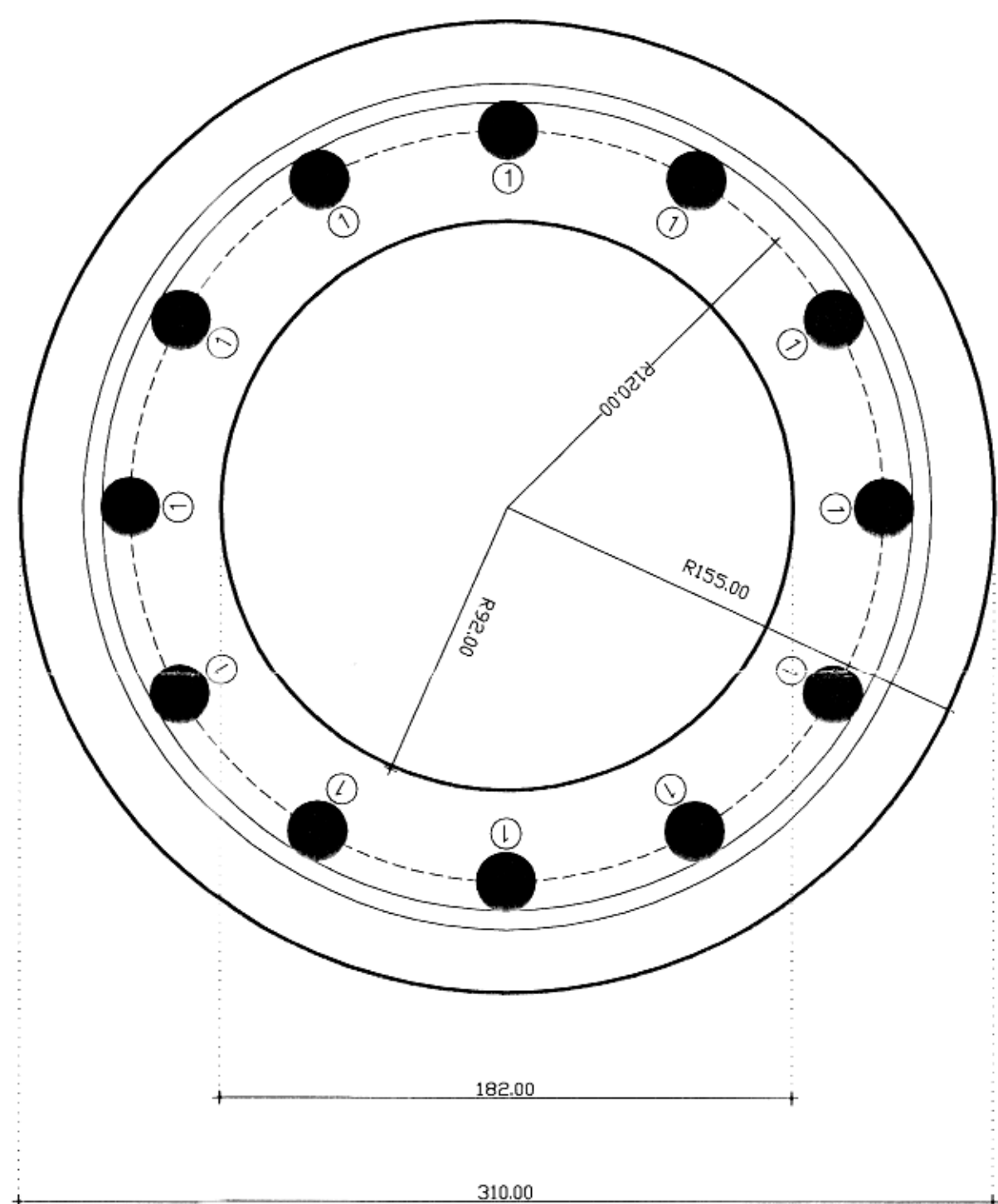
ΤΙΜΕΝΤΟΣΤΥΛΟΣ ΕΒ11 ΤΟΜΗ Β-Β ΔΙΑΤΑΞΗ ΟΠΤΑΣΜΟΥ ΚΕΦΑΛΗ ΣΤΥΛΟΥ ΚΑΙΜΑΚΑ 1:2
